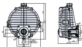
CR 1:5,9 Ø 3/4" cod.1666
