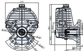
CR 1:5,9 Ø 1" cod.33261
