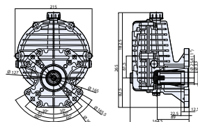
CR 1:5,9 Ø 1" cod.33261
