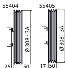
Puleggia Pulley
