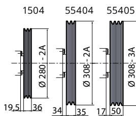
Puleggia Pulley
