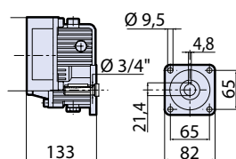
CR 1:5,9 Ø 3/4" cod.1636
