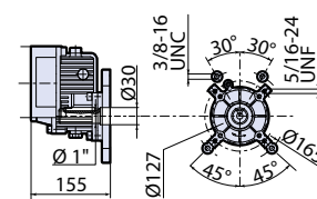
CR 1:5,9 Ø 1" cod.1639
