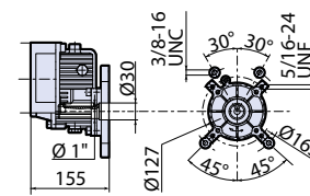
CR 1:5,9 Ø 1" cod.1639
